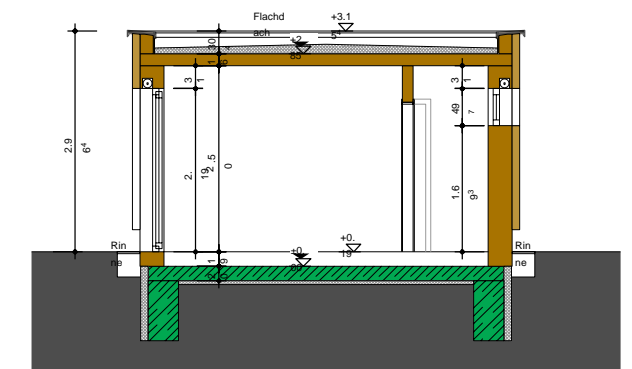
SCHNITT A-A Flachdach-Holzschalung
