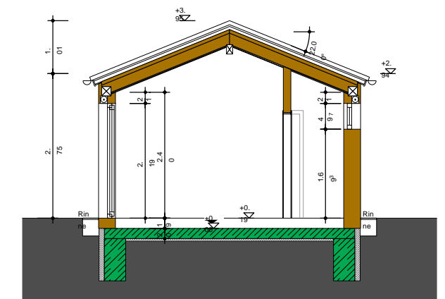
SCHNITT A-A Satteldach
