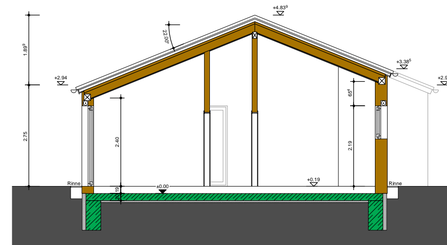
SCHNITT A-A Satteldach
