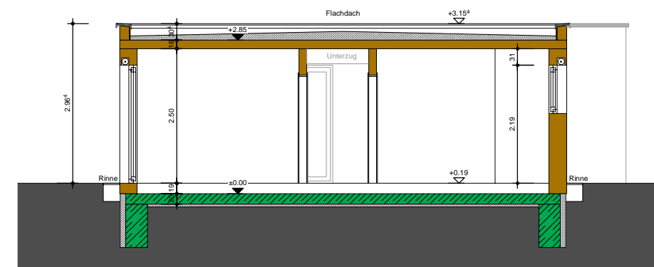
SCHNITT A-A Flachdach
