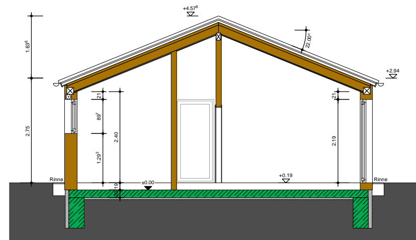
SCHNITT A-A Satteldach
