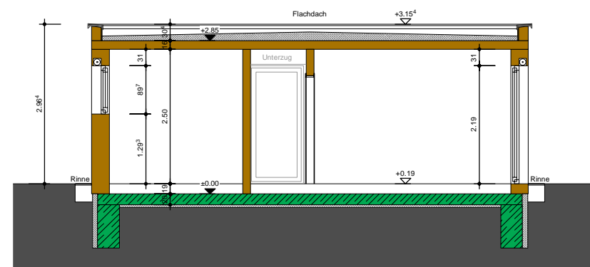
SCHNITT A-A Flachdach
